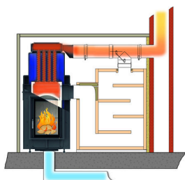
Gebruik van de ketel met Moritz-klep
