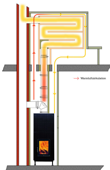
Bijkomende optie set rookkanaalaansluitingen in plaats van Moritz-klep
