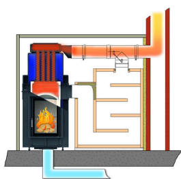
Gebruik van de ketel met Moritz-klep
