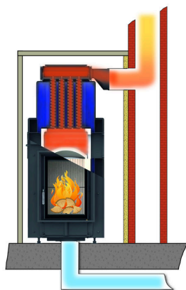
Gebruik van de ketel met directe aansluiting
