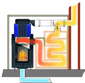
Opslag met Moritz-klep
