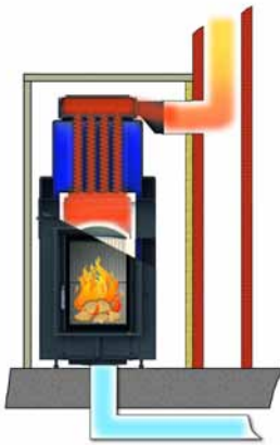
Gebruik van de ketel met directe aansluiting
